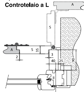
Monoblocco Apertura a Libro Controtelaio a L
