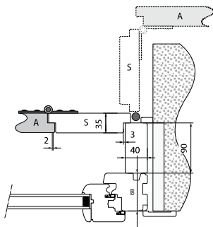
Monoblocco Apertura a Libro
