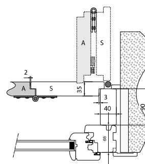
Monoblocco Apertura a Pacchetto
