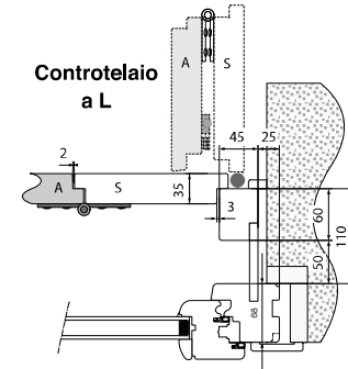
Monoblocco con Zanzariera Apertura a Pacchetto
