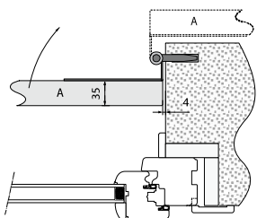
A Murare con Bandella Zancata
