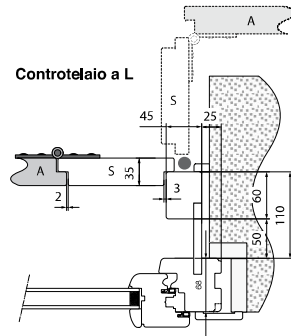
Monoblocco con Zanzariera Apertura a Libro
