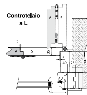
Monoblocco Apertura a Pacchetto
