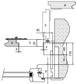
Monoblocco con Zanzariera Apertura a Libro
