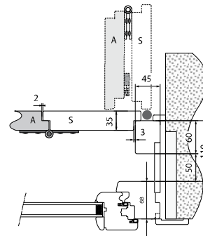
Monoblocco con Zanzariera Apertura a Pacchetto
