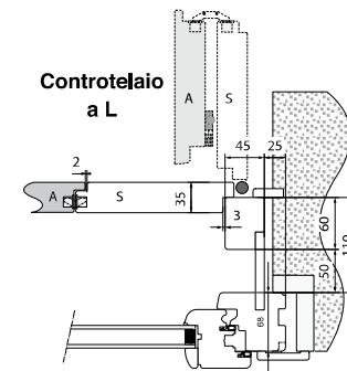
Versione con Cerniere a Scomparsa
