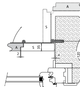
A Murare Apertura a Libro
