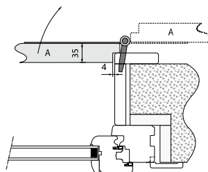
Esterno Muro con Telaio in Legno
